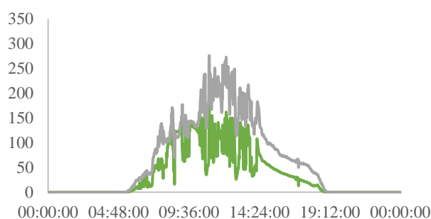
Figure 7 Evolution journalière du rayonnement global au point de mesure 1,8m sur façade végétalisée (vert) et sur une façade minérale (gris) orientation Nord
