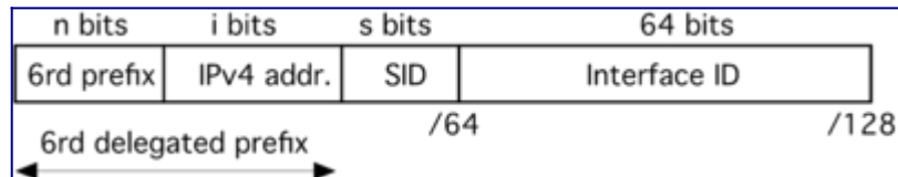
Figure 12 : Format d'une adresse 6rd .
