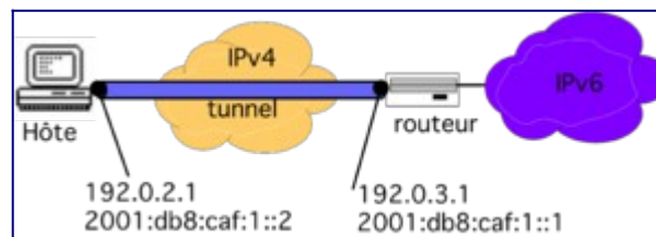
Figure 4 : Cas d'un tunnel configuré.
