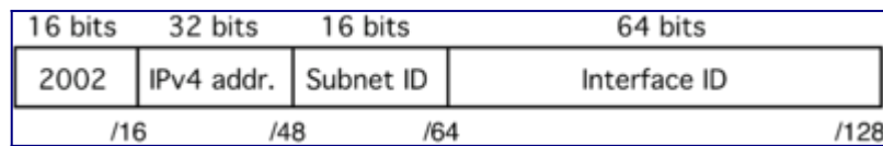
Figure 9 : Format d'une adresse construite sur la base d'une connectivité par un tunnel.
