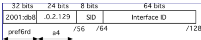
Figure 13 : Exemple de construction d'un préfixe délégué 6rd .
