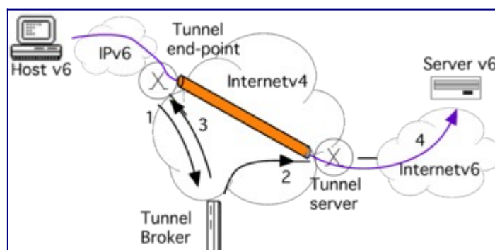
Figure 6 : Configuration d'un Tunnel Broker avec TSP.
