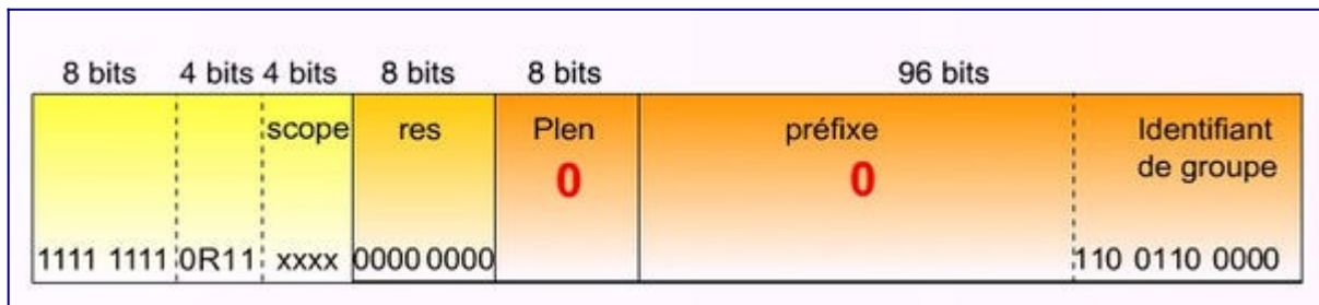
Figure 6 : Format de l'adresse multicast SSM.
