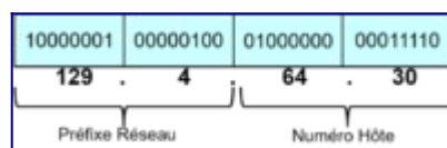
Figure 4 : Notation de l'adresse réseau en décimal.
