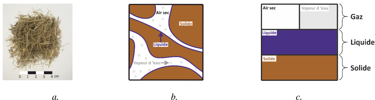
Figure 2 : La bagasse réelle (a), schématisée en présence des 3 phases (b) et la représentation moyennée (c).
