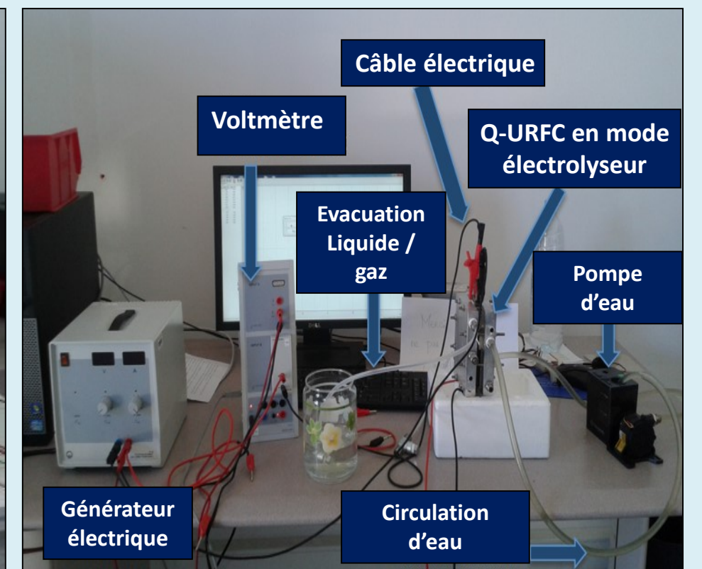
Banc de tests pour Electrolyseurs PEM (montage laboratoire)
