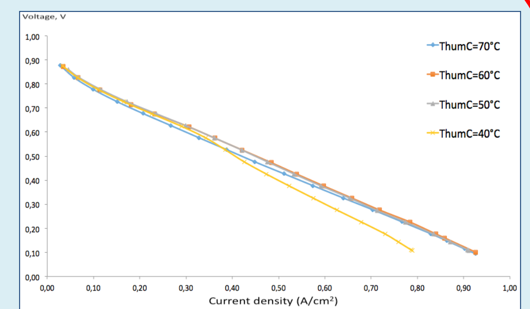
Courbes de polarisation en mode-PAC pour différents Température d'humidification cathodique de la Q-URFC ( S_{act} = 26 \text{ cm}^2 , T_{cell} = T_{hum,A} = 75^\circ \text{ C} , P = 1 \text{ Bar} , Q_{H_2} = 400 \text{ ml/min} , Q_{O_2} = 200 \text{ ml/min} ).
