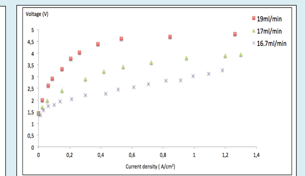
Courbes de polarisation en mode-E pour différents débits d'eau de la Q-URFC ( S_{act} = 16 \text{ cm}^2 , P = 1 \text{ Bar} , T_{cell} = 60^\circ \text{ C} ).
