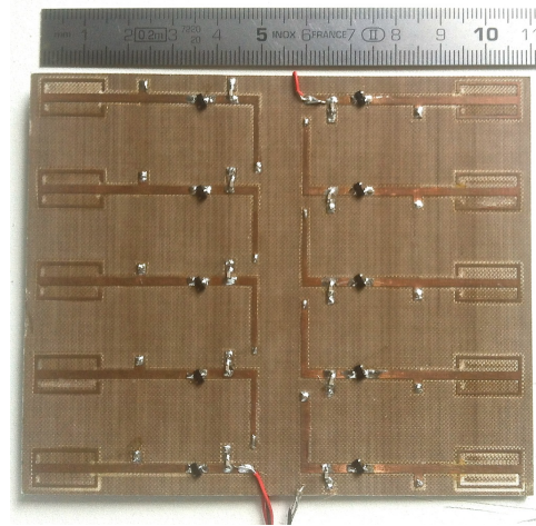
Fig. 5. Rectenna array
