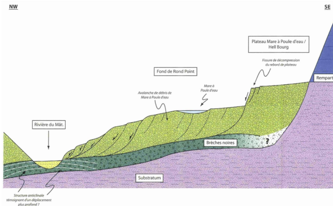
Figure 5: Coupe géologique schématique et interprétative du glissement de Mare à Poule d'Eau. D'après Garnier et Lucas, 2008. Attention, les axes verticaux et horizontaux ne sont pas la même échelle.
