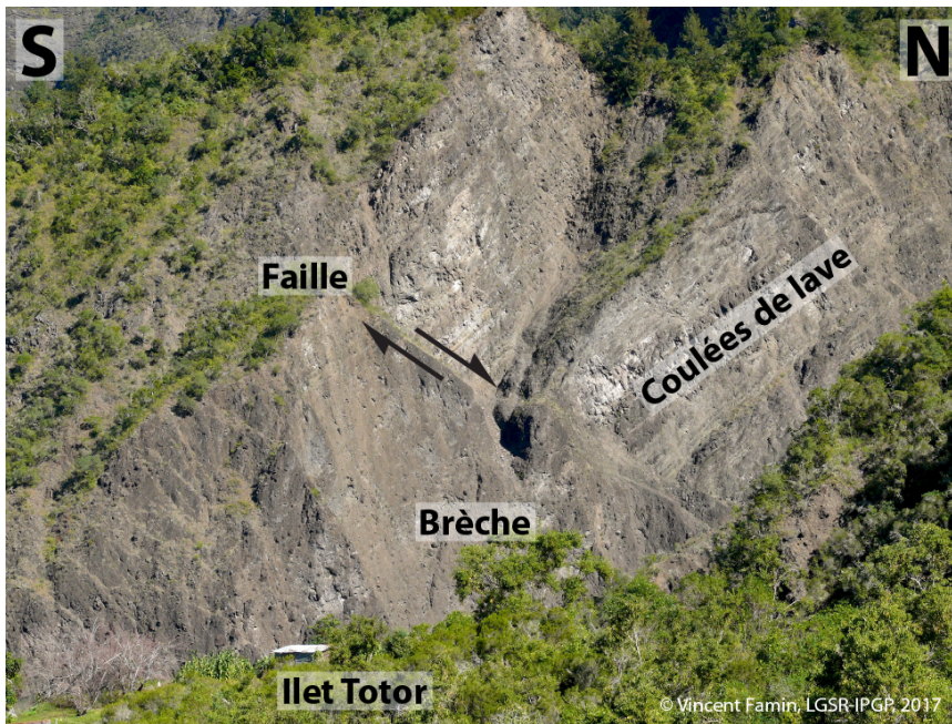
Figure 3 : Zoom sur la faille qui juxtapose les coulées de lave du Tapcal et la brèche sous-jacente, vue depuis le point d'observation N°1. Photo: Vincent Famin.
