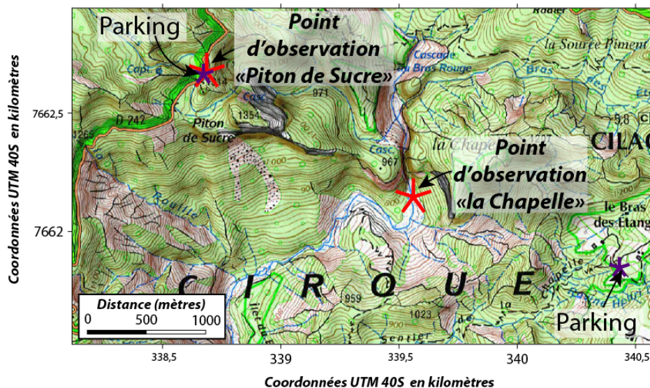
Figure 1: Localisation des deux points d'observation de la syénite du Piton de la
