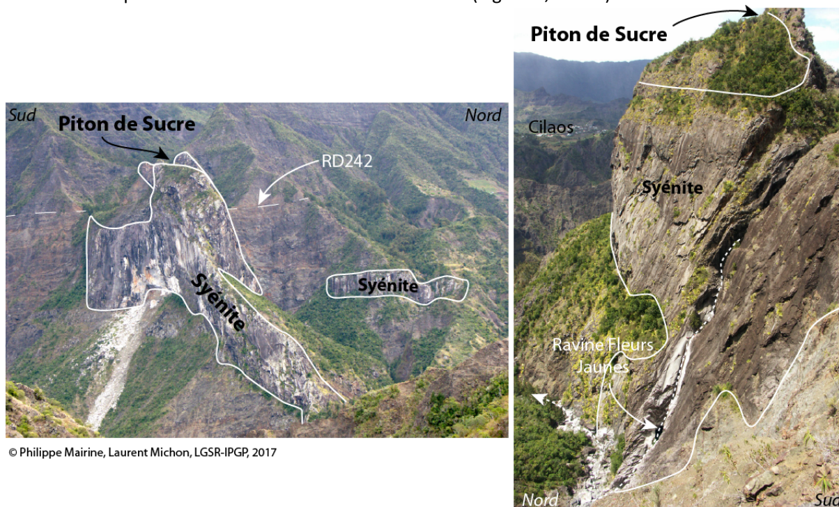
Figure 3: Gauche: Vue de l'intrusion du Piton de Sucre depuis Cilaos. Cette intrusion présente un pendage vers le Nord qui tend à s'horizontaliser dans la zone de la Chapelle. Droite: Syénite du Piton de Sucre depuis le point d'observation. Photos: Philippe Mairine.
