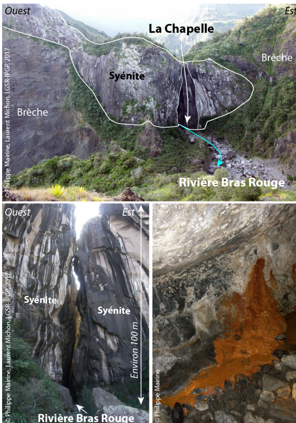
Figure 4: Haut: Panorama sur le site de la Chapelle depuis le sentier d'accès. L'intrusion est injectée dans des brèches antérieures du Piton des Neiges, datant de sa période basique, avant 430 ka). La rivière de Bras Rouge a incisé la syénite sur toute son épaisseur. Bas à gauche: Canyon incisé par la rivière du Bras Rouge. Bas à droite: Source thermo-minérale émergeant au sein de la syénite dans le canyon. La couleur orange indique la forte teneur en fer de cette eau thermique. Photos: Philippe Mairine.
